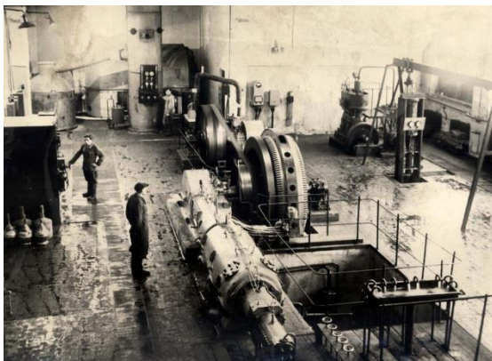
Рис. 4. Внутренний вид цеха жидкого кислорода Оксидквритного завода. 1940-е гг.
